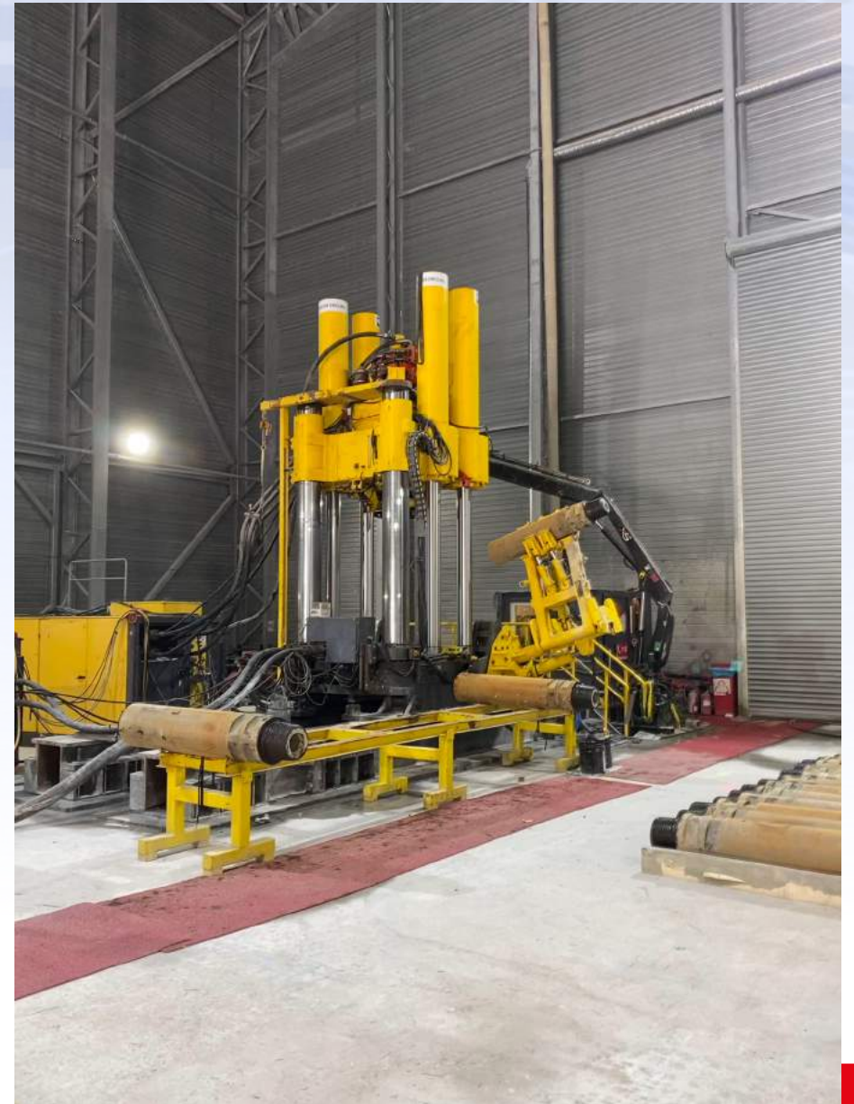
Forage du trou pilote pour raise-boring
